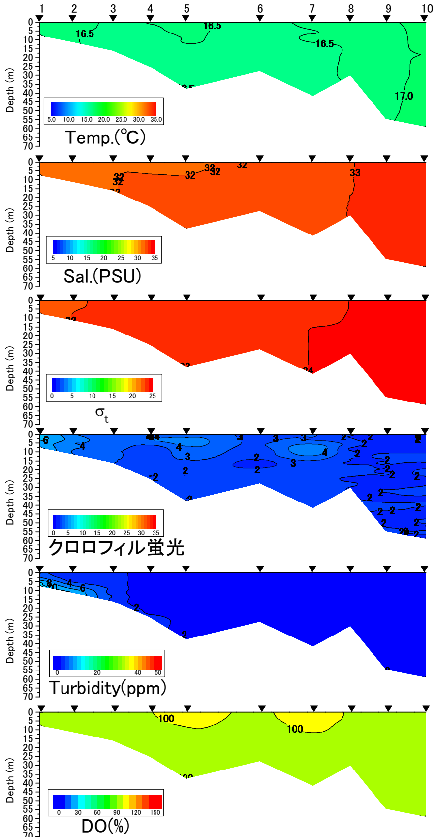
有明海中央ラインの水温(°C)、塩分、密度( \sigma_t )、クロロフィル蛍光強度、濁度、溶存酸素飽和度(DO%)の鉛直面図(国土交通省の調査による) (2014年4月30日)
